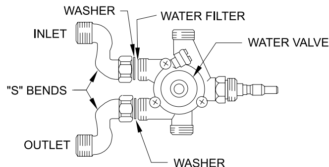
Vanne manométrique et raccords "S" - vue de dessus
