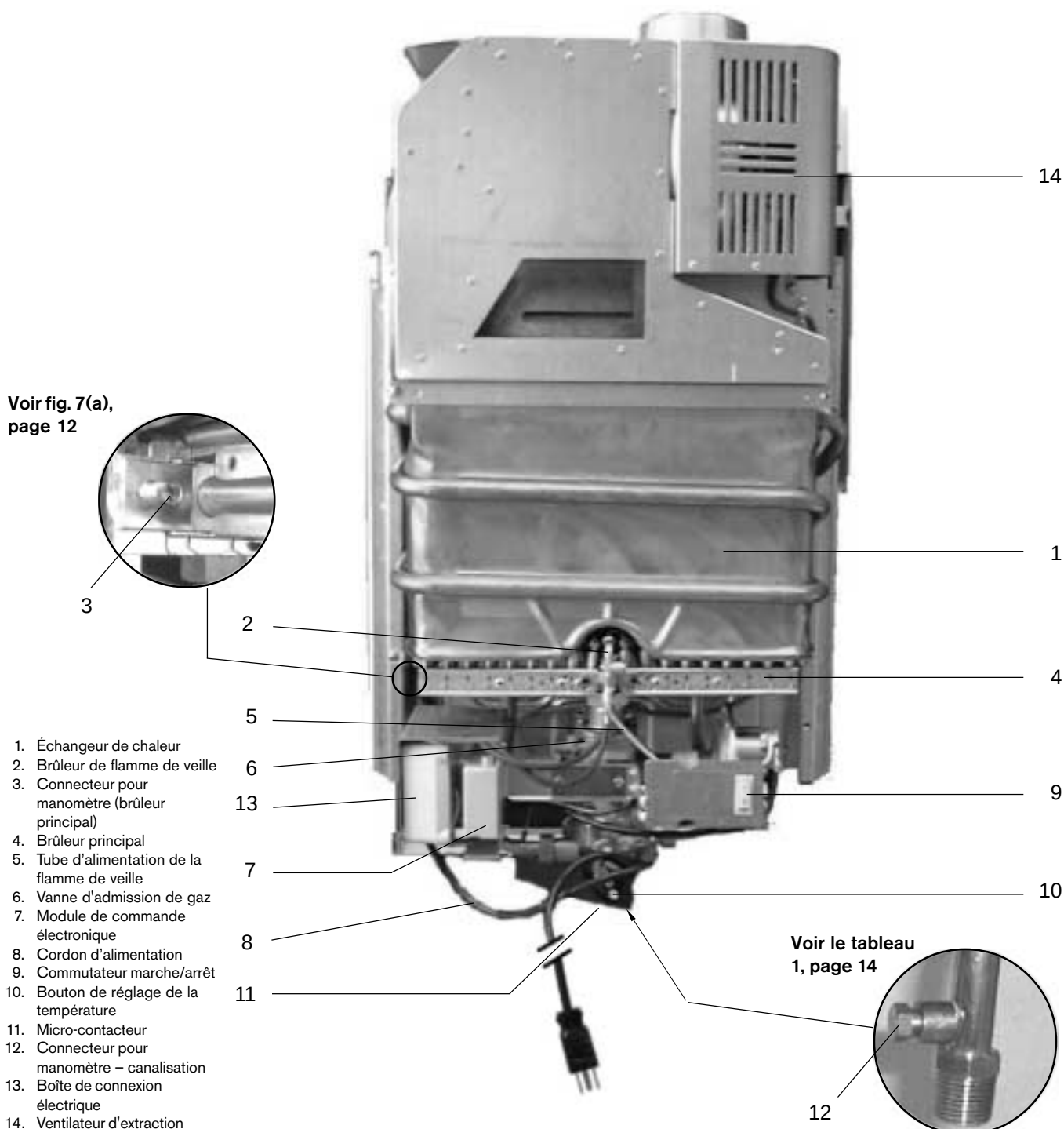
Fig. 17 - Chauffe-eau WR430-3K
