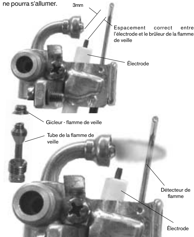
Fig. 13 - Dispositif de la flamme de veille
